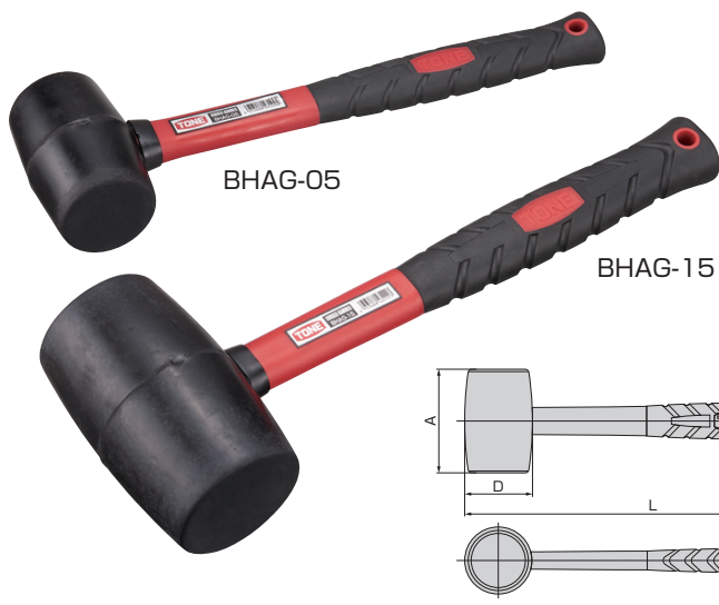
■寸法図
