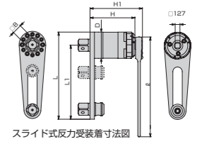
スライド式反力受装着寸法図
