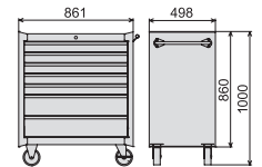
■ WSW207R ワイドローラーキャビネット寸法
