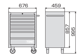
WS207R(S)(B)ローラーキャビネット寸法
