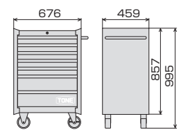
WS207R(S)(B)ローラーキャビネット寸法
