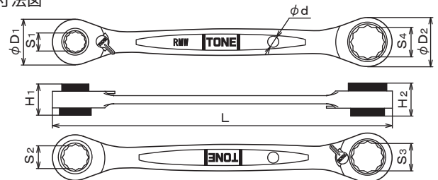
※外觀寸法図
