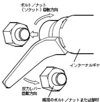
③ソケットを差し込む
