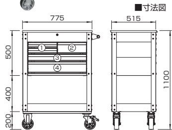
■寸法図
