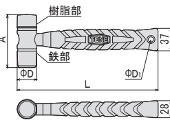
■寸法図
