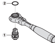
RH3VHS 部品展開図
